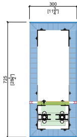
INNER FIN
