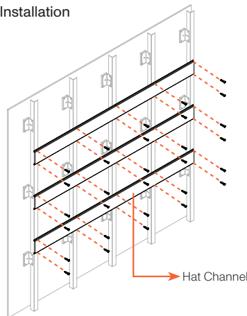
Hat Channel
