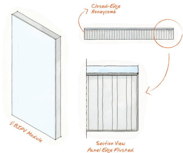
Module Edge Flushed
