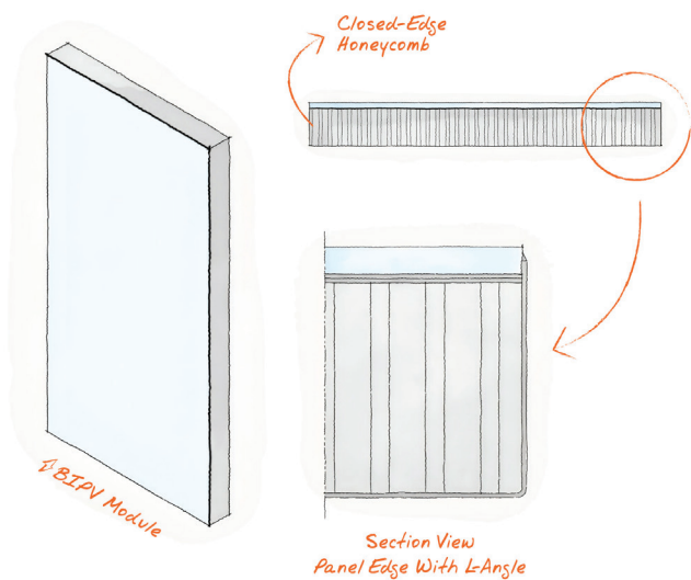
Module Edge With L-Angle
